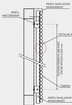
DETALHES DE INSTALAÇÃO BRISE HORIZONTAL
